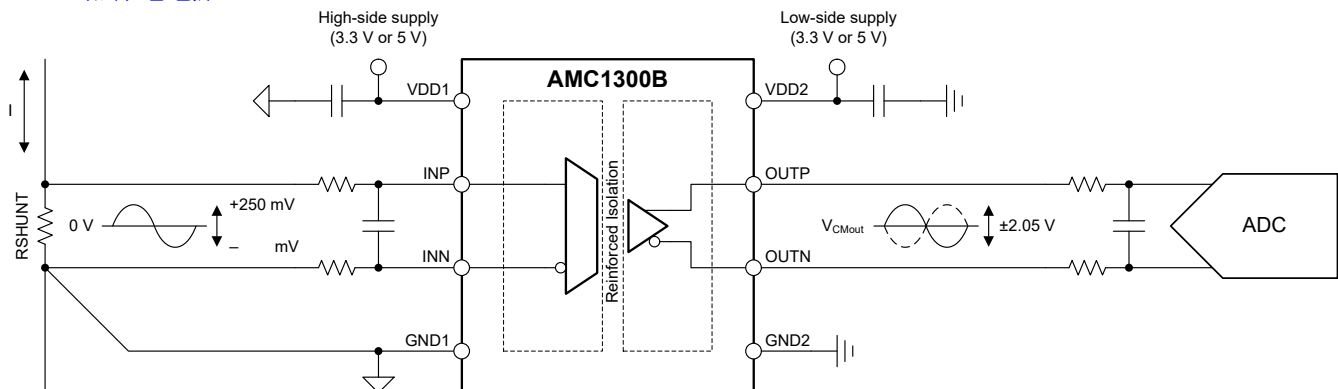
概略回路図
