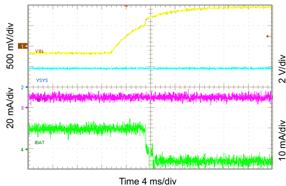
10-7. OVP Fault
