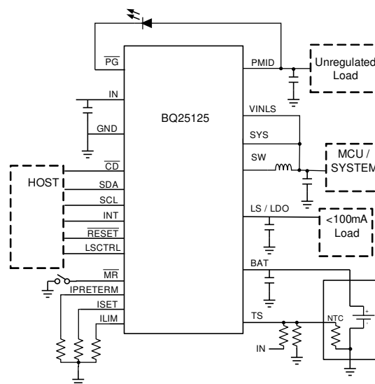
概略回路図
