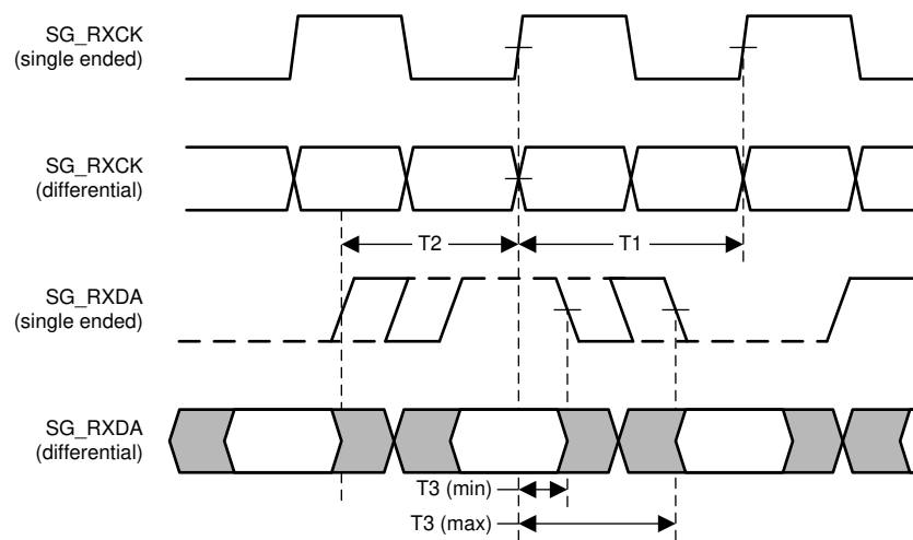
图 6-4. SGMII Timing
