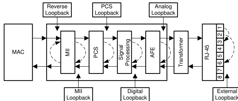
図 7-9. Loopbacks
