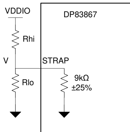
図 7-10. Strap Circuit
