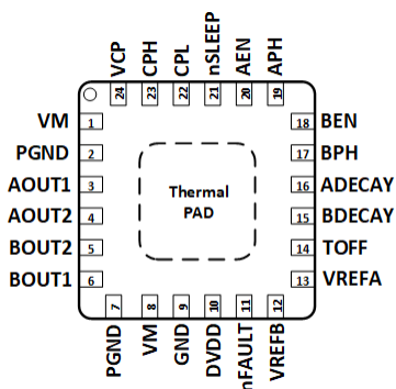
図 5-2. RGE パッケージ 24 ピン VQFN (露出サーマル・パッド付き) 上面図 DRV8426E
