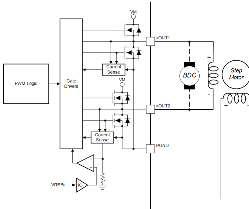
図 7-4. PWM モータ・ドライバのブロック図
