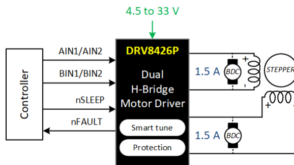
DRV8426P の概略回路図
