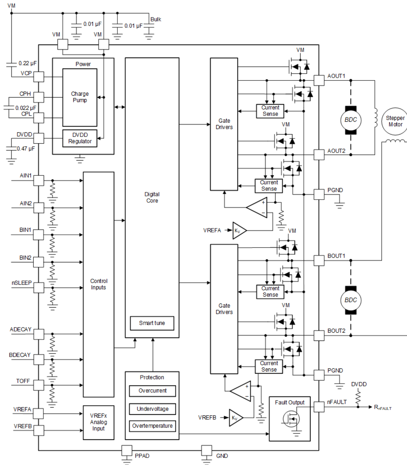
図 7-2. DRV8426P のブロック図
