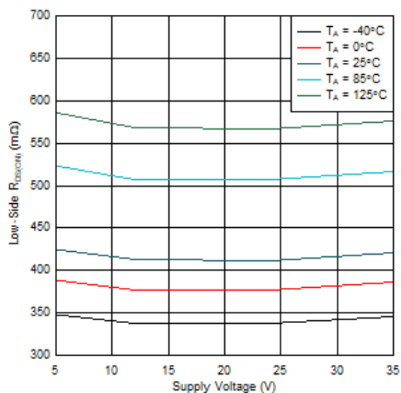
図 6-5. ローサイド R_{DS(ON)} と電源電圧
