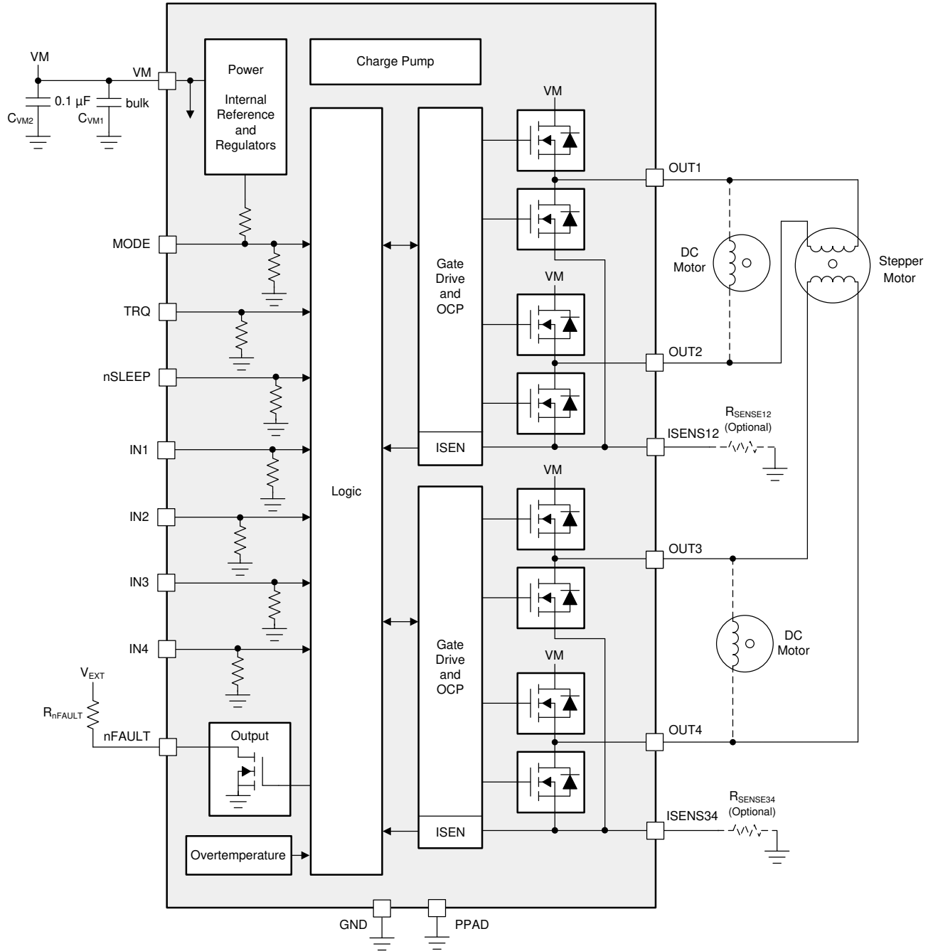
図 7-1. DRV8847 のブロック図
