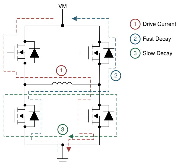
図 7-12. 減衰モード
