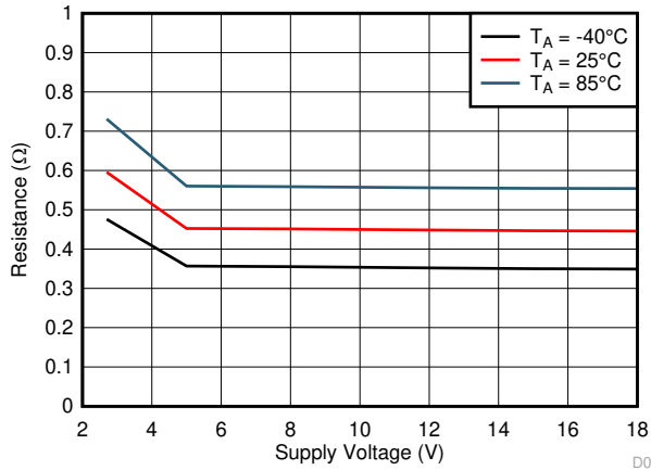
図 6-9. ローサイド オン抵抗 ( R_{DS(ON)_LS} ) と電源電圧 ( V_{VM} ) との関係
