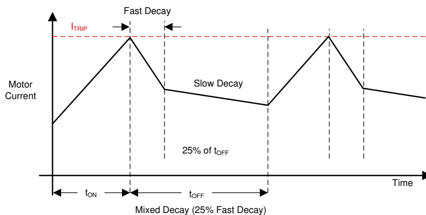
図 7-13. 混合減衰
