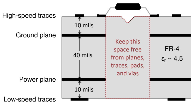
✎ 8-6. Layout Example
