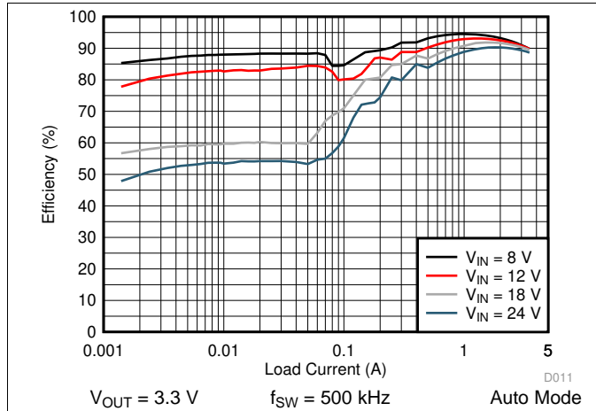
图 23. LM76003 Efficiency
