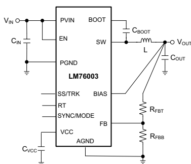
概略回路図
