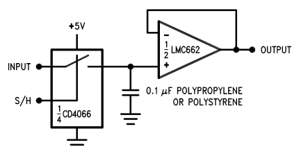
代表的なアプリケーション：低リークのサンプル / ホールド
