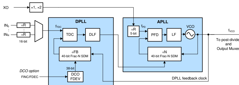
図 3-1. 対になった DPLL と APLL のブロック図
