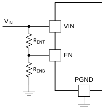
图 35. System UVLO
