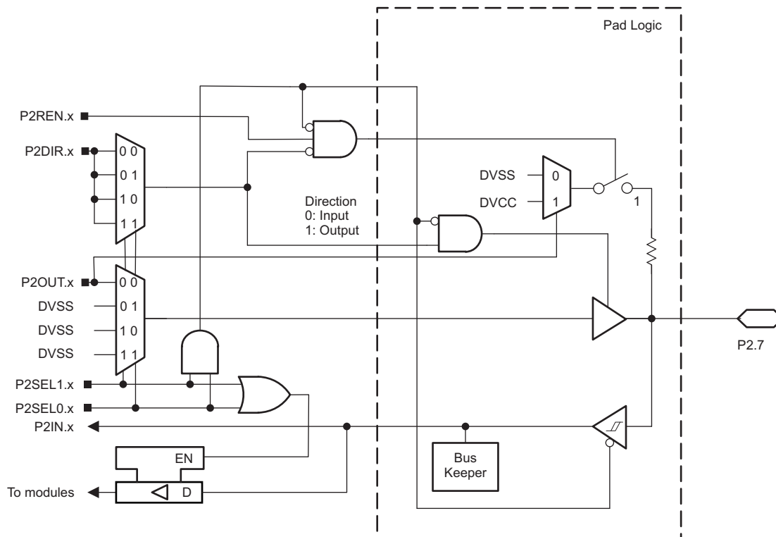
☒ 6-9. Port P2 (P2.7) Diagram
