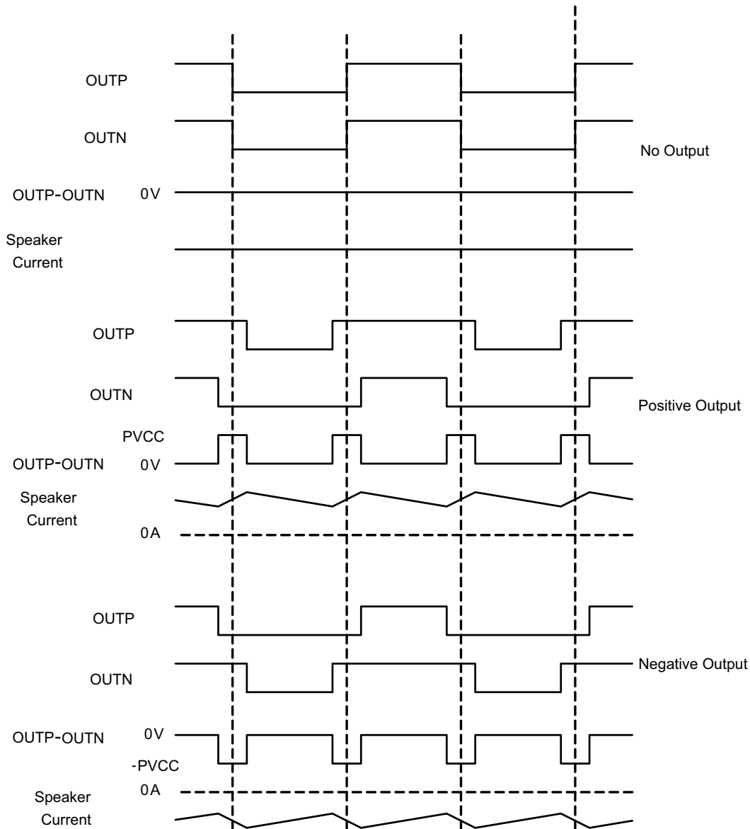
FIG 9-8. BD Mode Modulation
