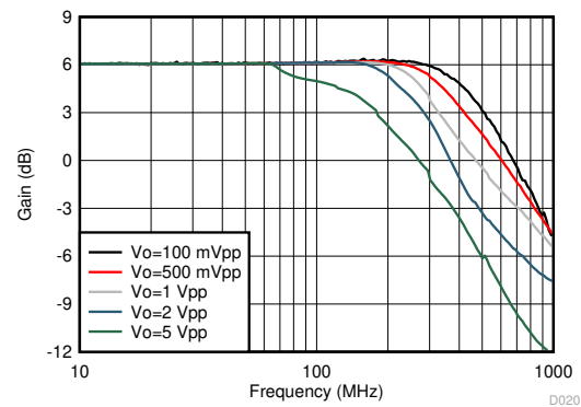
図 7-1 を参照、 V_{CC} = 3V 、 V_{ocm} = 1.5V
