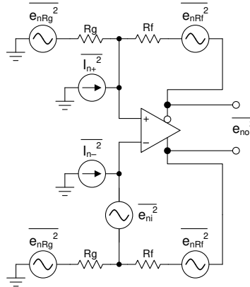
図 7-10. FDA ノイズ解析回路
