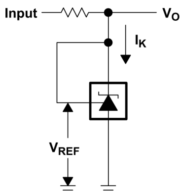
6-1. Test Circuit for v_{KA} = V_{REF} , V_O = V_{KA} = V_{REF}
