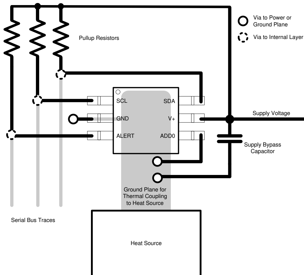
图 7-4. TMP102 Layout Example
