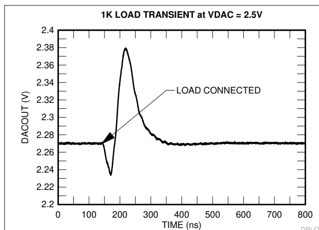
図 7-55. 1k \Omega の負荷過渡応答
