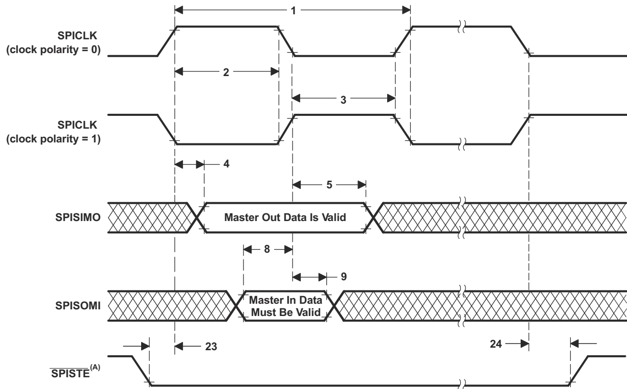
図 7-88. 高速 SPI マスタ・モードの外部タイミング (クロック位相 = 0)
