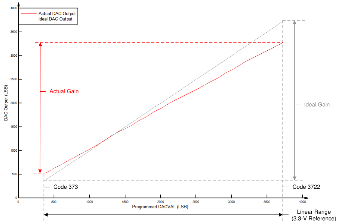
図 7-49. バッファ付き DAC のゲイン
