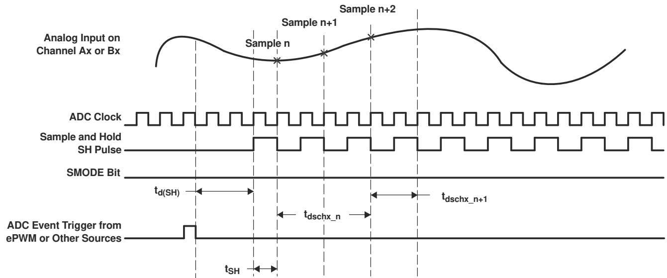
図 7-39. シーケンシャル・サンプリング・モード (シングル・チャンネル) のタイミング
