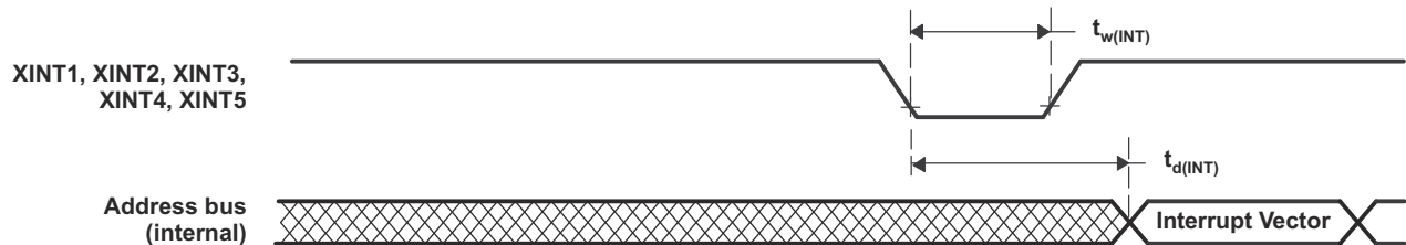
図 6-20. 外部割り込みのタイミング
