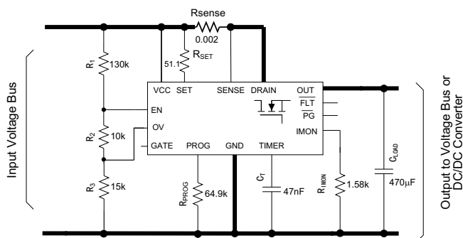
アプリケーション回路図 (12V、10A)
