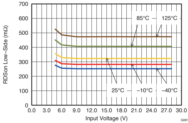
図 29. ローサイド・スイッチ
