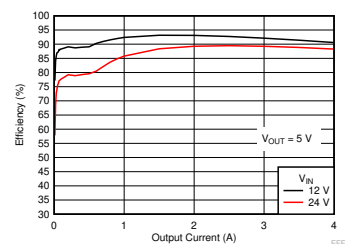
5V OUT の効率
