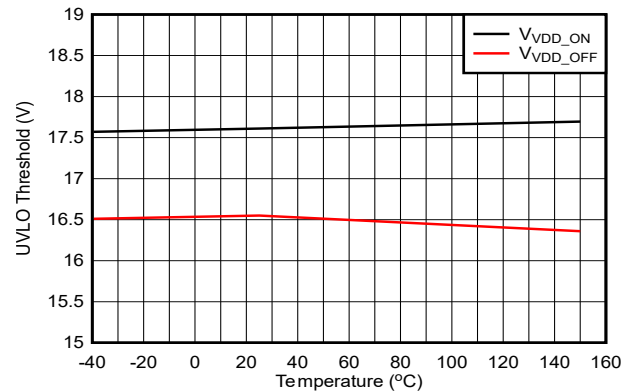
図 5-21. VDD 17V UVLO スレッシュホールドと温度との関係
