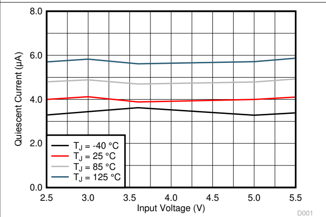
图 6-4. Quiescent Current
