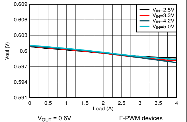
図 8-6. Load Regulation
