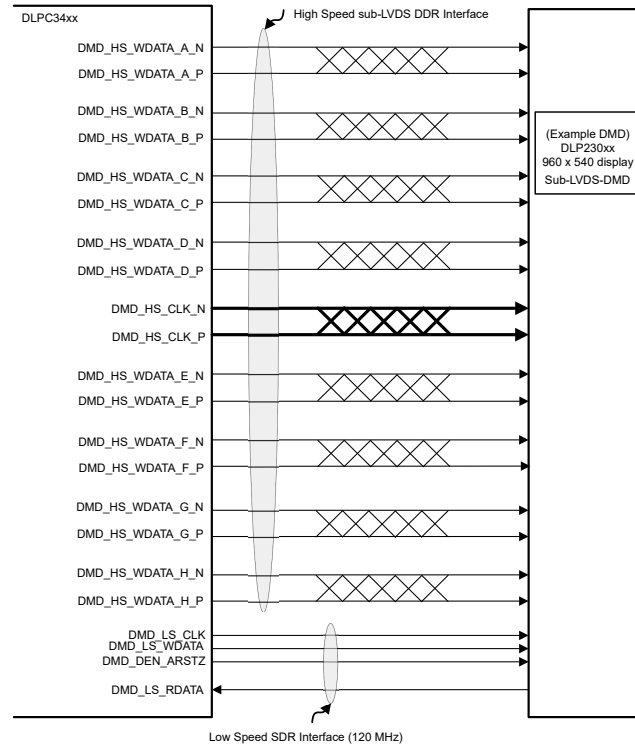
FIG 7-11. DLP230NP/NPSE (.23 Full HD) DMD Interface Example
