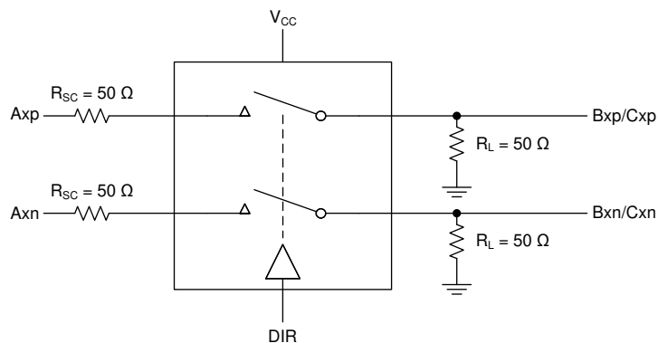
図 6-1. テスト構成
