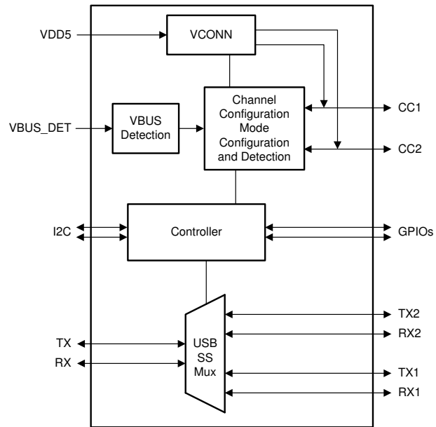
概略回路図
