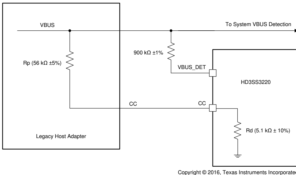
図 7-1. レガシー・アダプタ実装回路
