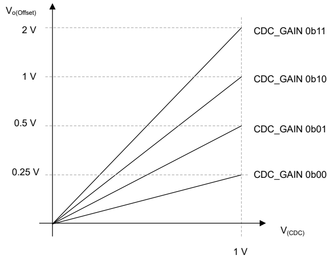
图 8-25. Vo Offset vs. CDC voltage
