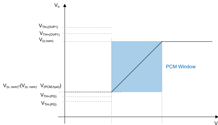
图 8-7. Output Voltage vs. Input Voltage
