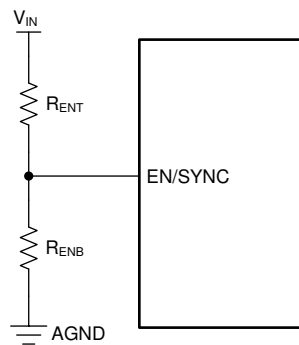
Figure 9-3. UVLO Using EN
