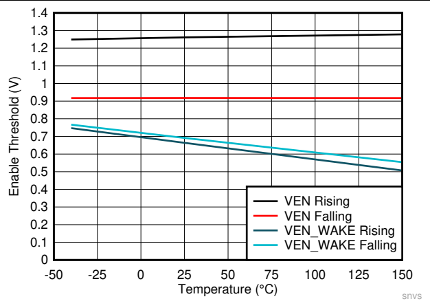
7-6. Enable Thresholds
