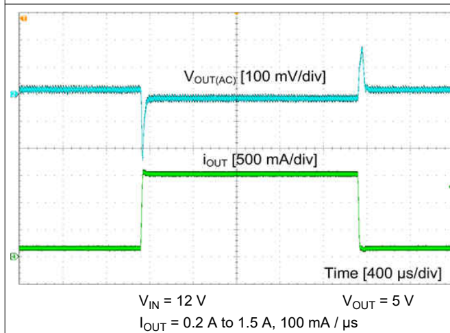
8-6. Load Transient
