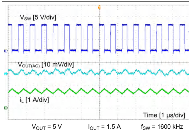
8-2. CCM Mode
