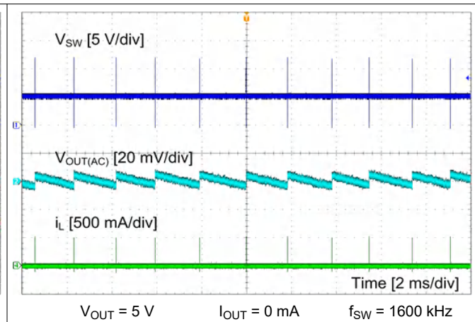
8-3. PFM Mode
