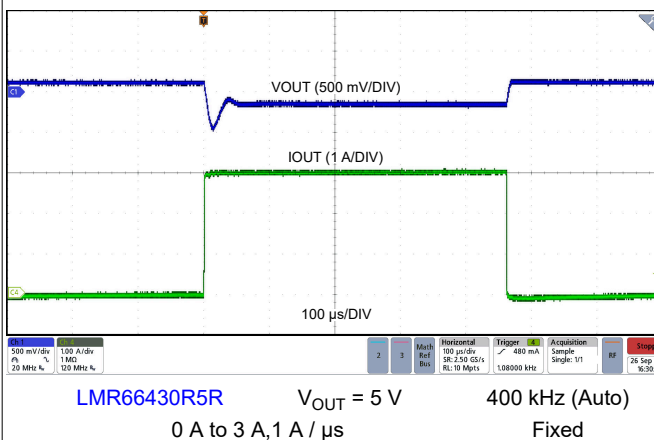
図 8-8. Load Transient
