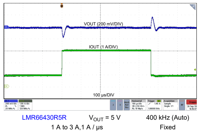
図 8-9. Load Transient
