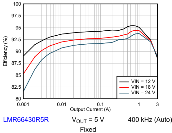
図 8-4. Efficiency
