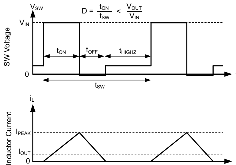
図 7-17. PFM Operation
