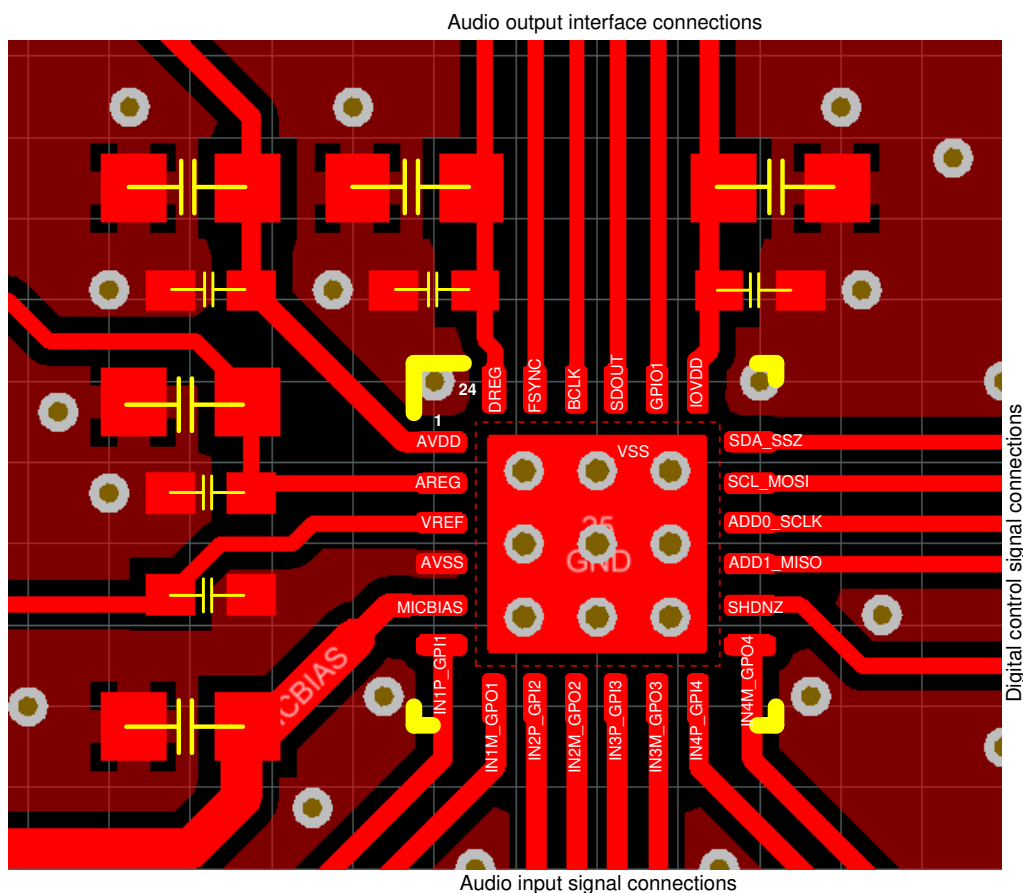
图 10-1. Layout Example
