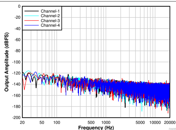
図 6-14. FFT With Idle Input
