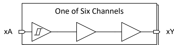
概略ロジック図
