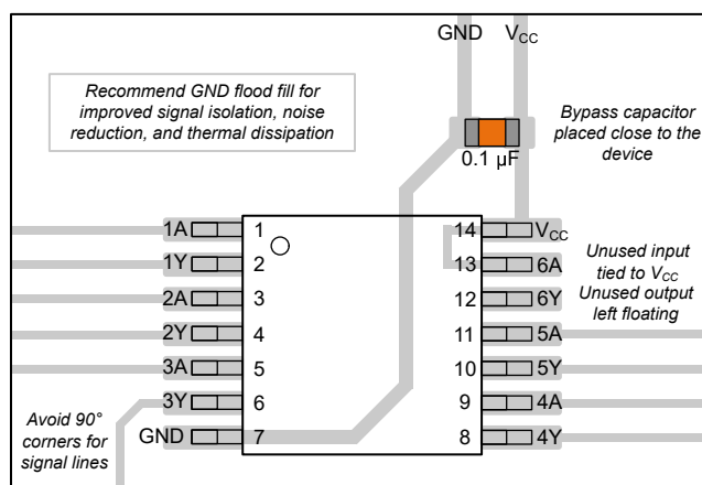
図 8-3. レイアウト例：SN54SC6T17-SEP
