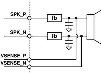
图 24. V-Sense Connections
