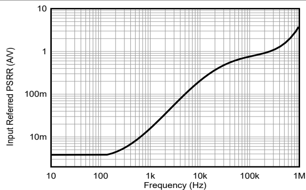
図 6-7. PSRR vs Frequency
