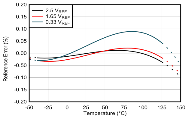
図 6-2. Reference Error vs Temperature
