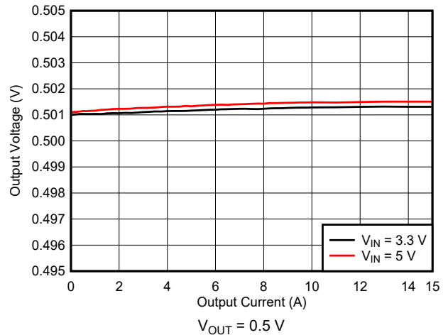
図 10-5. Load Regulation
