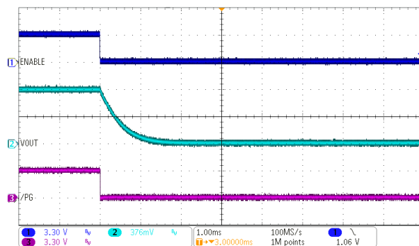
10-21. Shutdown Using the EN Pin (Discharge Enabled)
