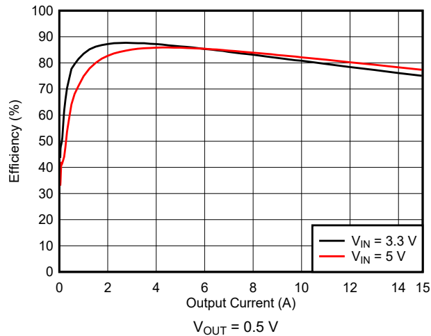
図 10-4. Efficiency
