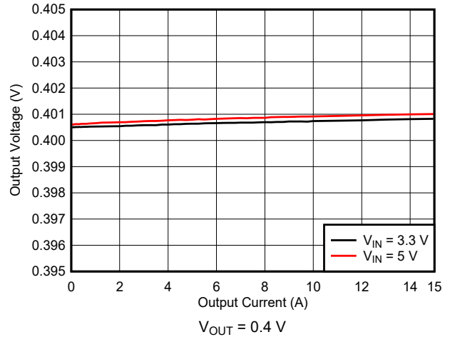
図 10-3. Load Regulation
