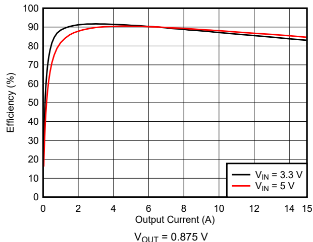
10-8. Efficiency
