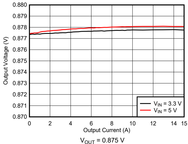
10-9. Load Regulation
