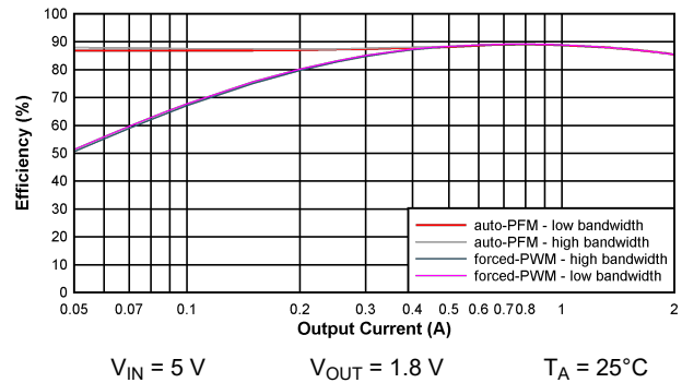
图 6-2. Efficiency BUCK23
