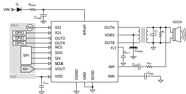
TUSS4440 アプリケーション図
