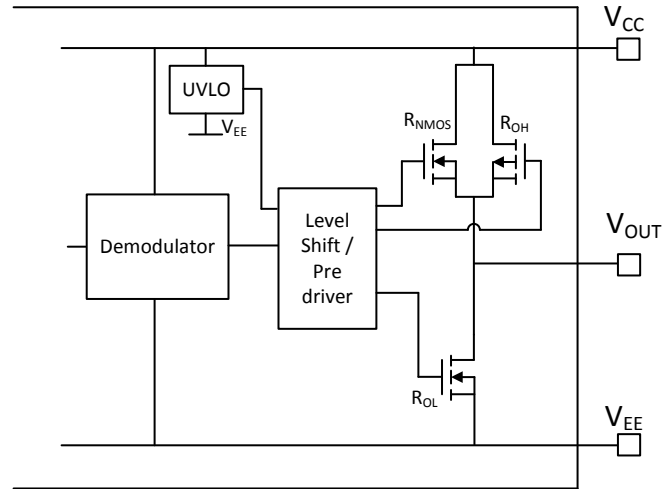
図 8-4. 出力段
