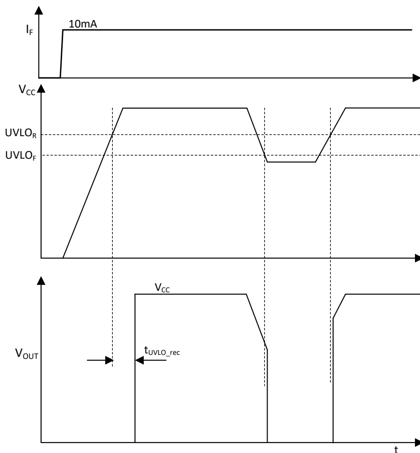
図 8-5. UVLO 機能
