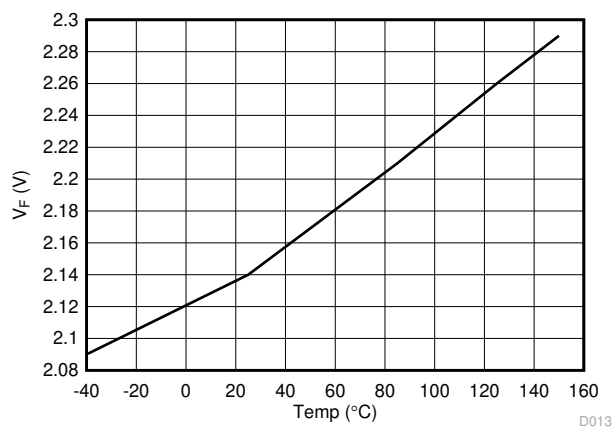
図 6-16. 順方向電圧降下と温度との関係
