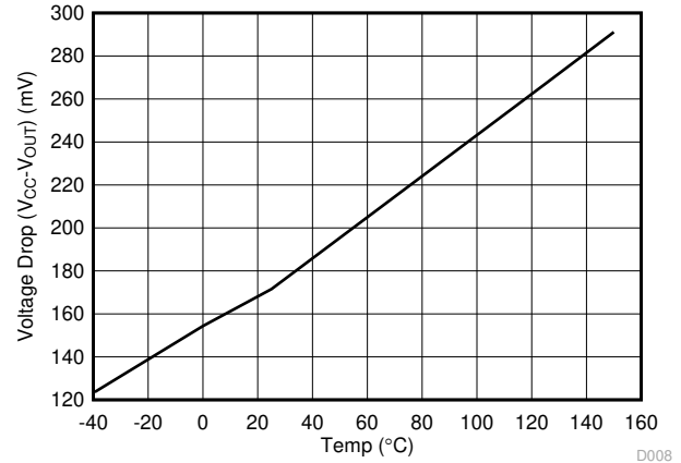
図 6-11. V_{OH} (20mA 負荷) と温度との関係
