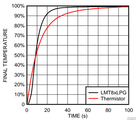
熱時定数
