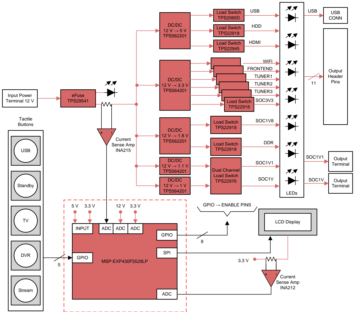
図 1. TIDA-01451 Block Diagram
