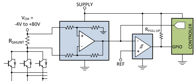
図 3. ハイサイドの過電流検出
