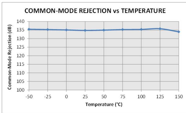
図 2. 動作温度に対するコモンモード除去性能
