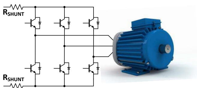
図 1. ローサイドとハイサイドの電流センシング
