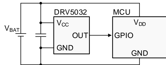
図 3. 一般的なマイクロコントローラの回路図
