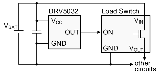
図 4. 一般的な負荷スイッチの回路図
