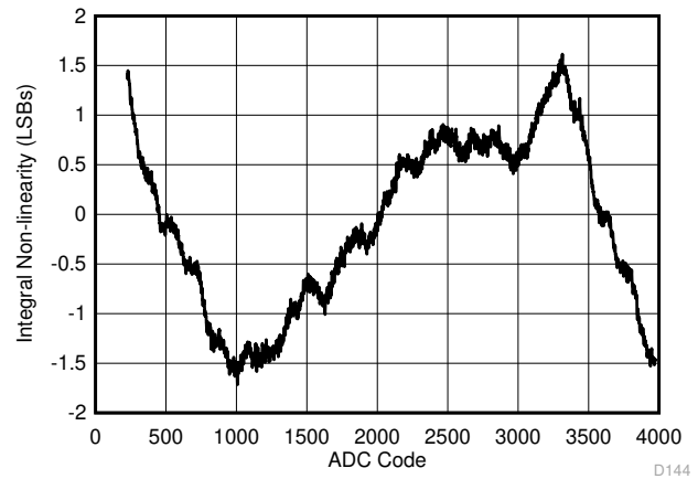
図 5-4. INL vs ADC Code
