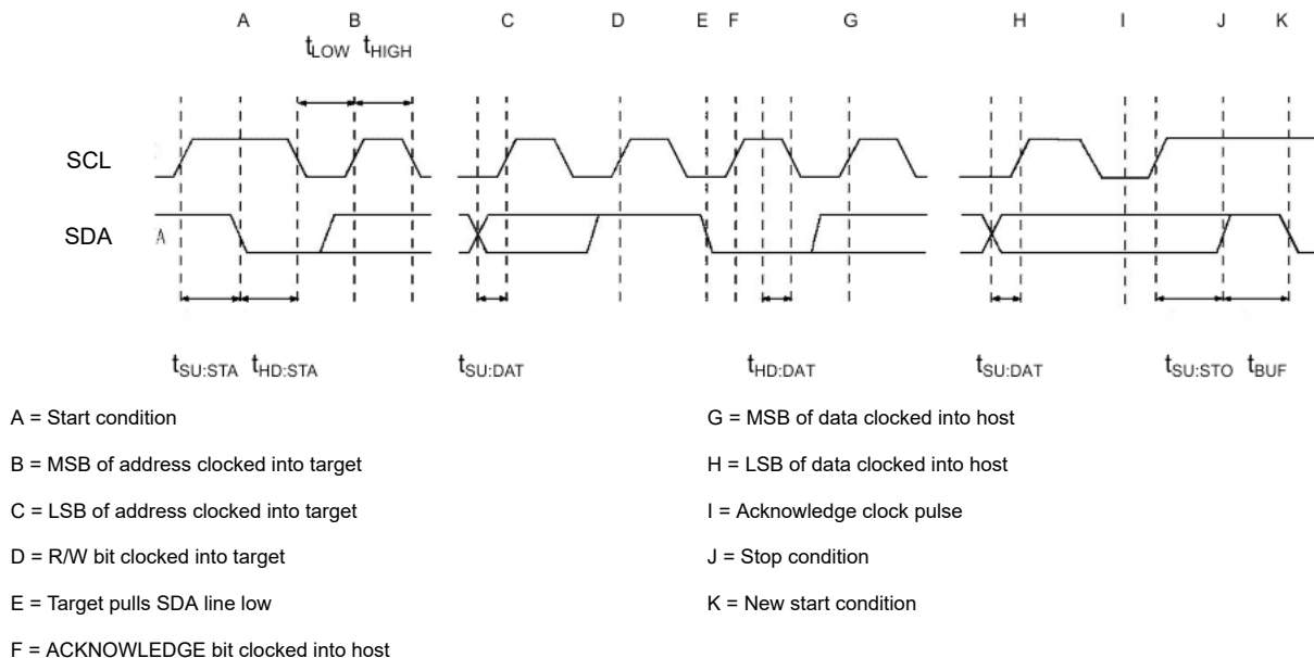
図 8-7. I 2 C Read Timing
