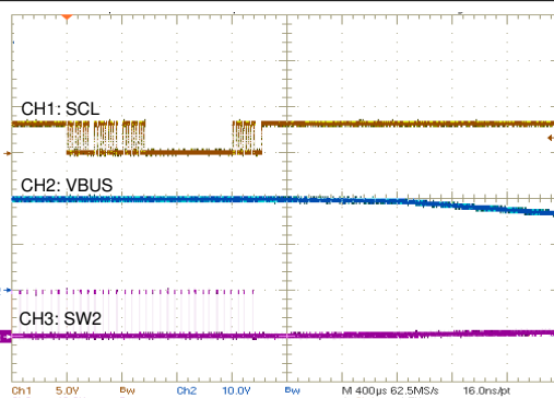
図 9-19. OTG Power Off
