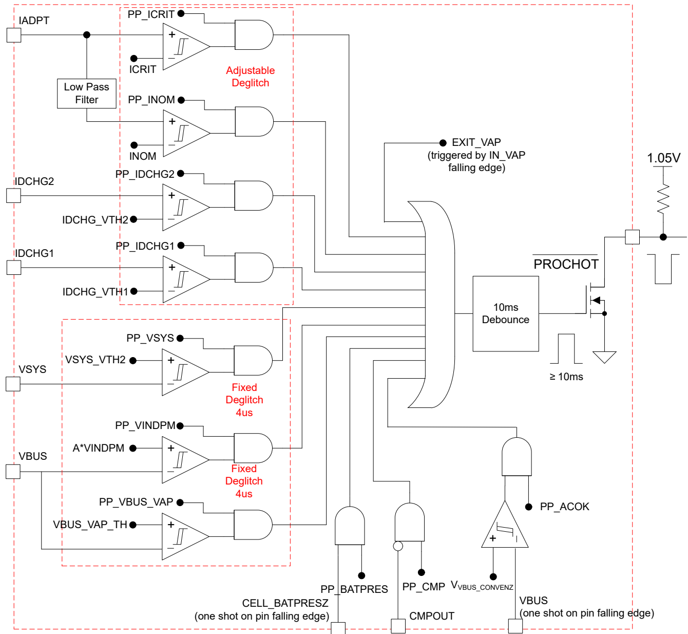
図 8-4. \overline{\text{PROCHOT}} Profile
