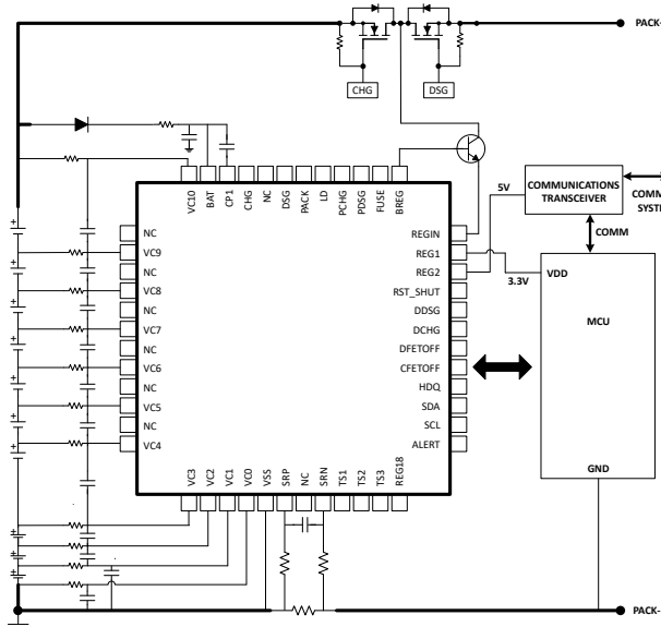
概略回路図
