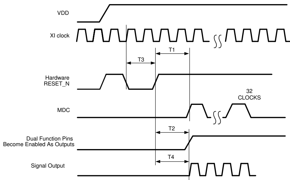
図 6-2. Reset Timing
