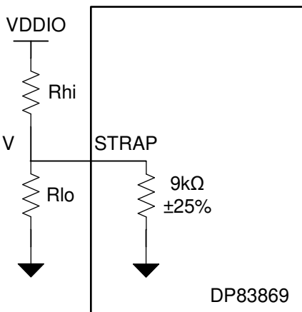
図 7-15. Strap Circuit
