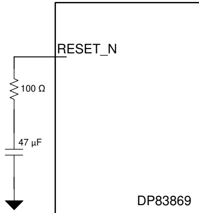
図 7-17. RESET_N Circuit
