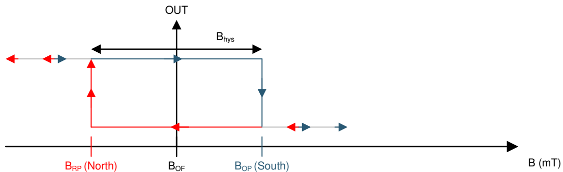
図 7-2. DRV5013-Q1 — B_{OP} > 0
