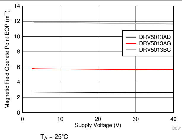
図 6-3. B_{OP} と V_{CC} との関係
