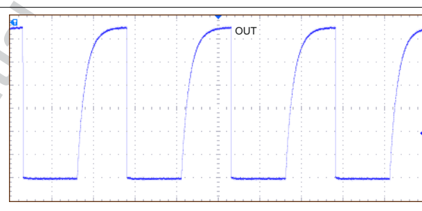
図 7-3. 10kHz のスイッチング磁界
