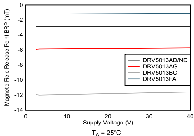
図 5-7. B_{RP} と V_{CC} との関係
