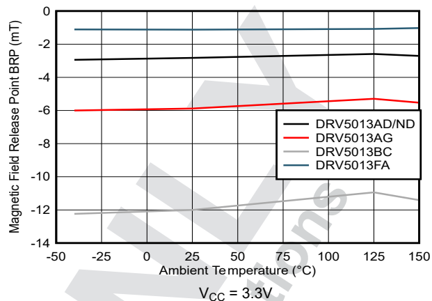
図 5-8. B_{RP} と温度との関係
