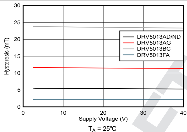
図 5-9. ヒステリシスと V_{CC} との関係
