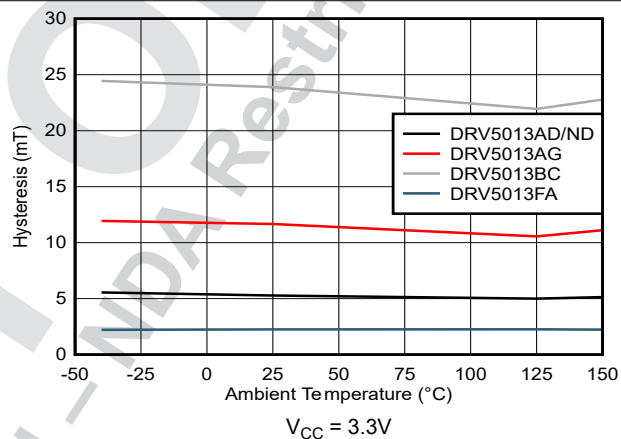
図 5-10. ヒステリシスと温度との関係
