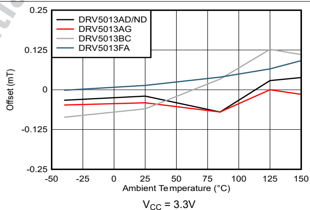
図 5-12. オフセットと温度との関係
