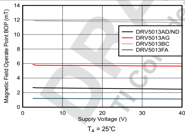
図 5-5. B_{OP} と V_{CC} との関係
