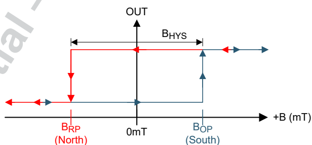
図 6-3. 反転出力状態 (ND バージョン)
