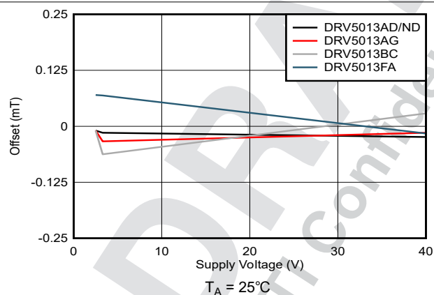
図 5-11. オフセットと V_{CC} との関係
