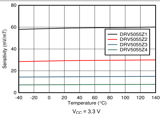
図 5-7. Sensitivity vs Temperature
