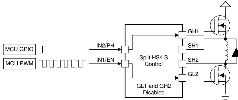
図 7-10. Solenoid Control Example
