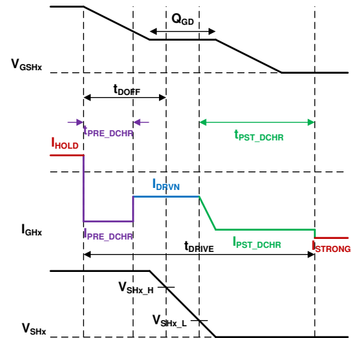
図 7-14. PDR Discharge Profile
