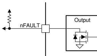
図 7-18. nFAULT ピン
