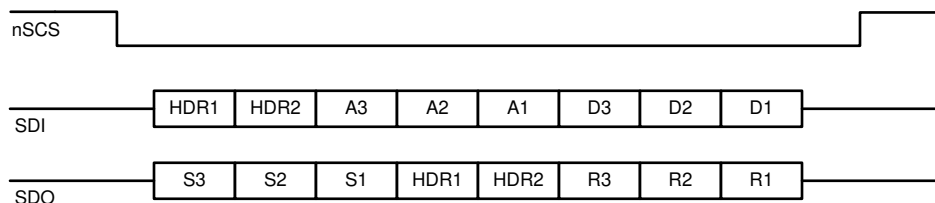
図 7-26. 3 つのデバイスのための SPI データ・シーケンス
