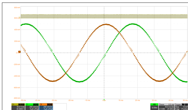
図 8-6. スマート・チューン・リップル制御減衰による 1/32 マイクロステッピング
