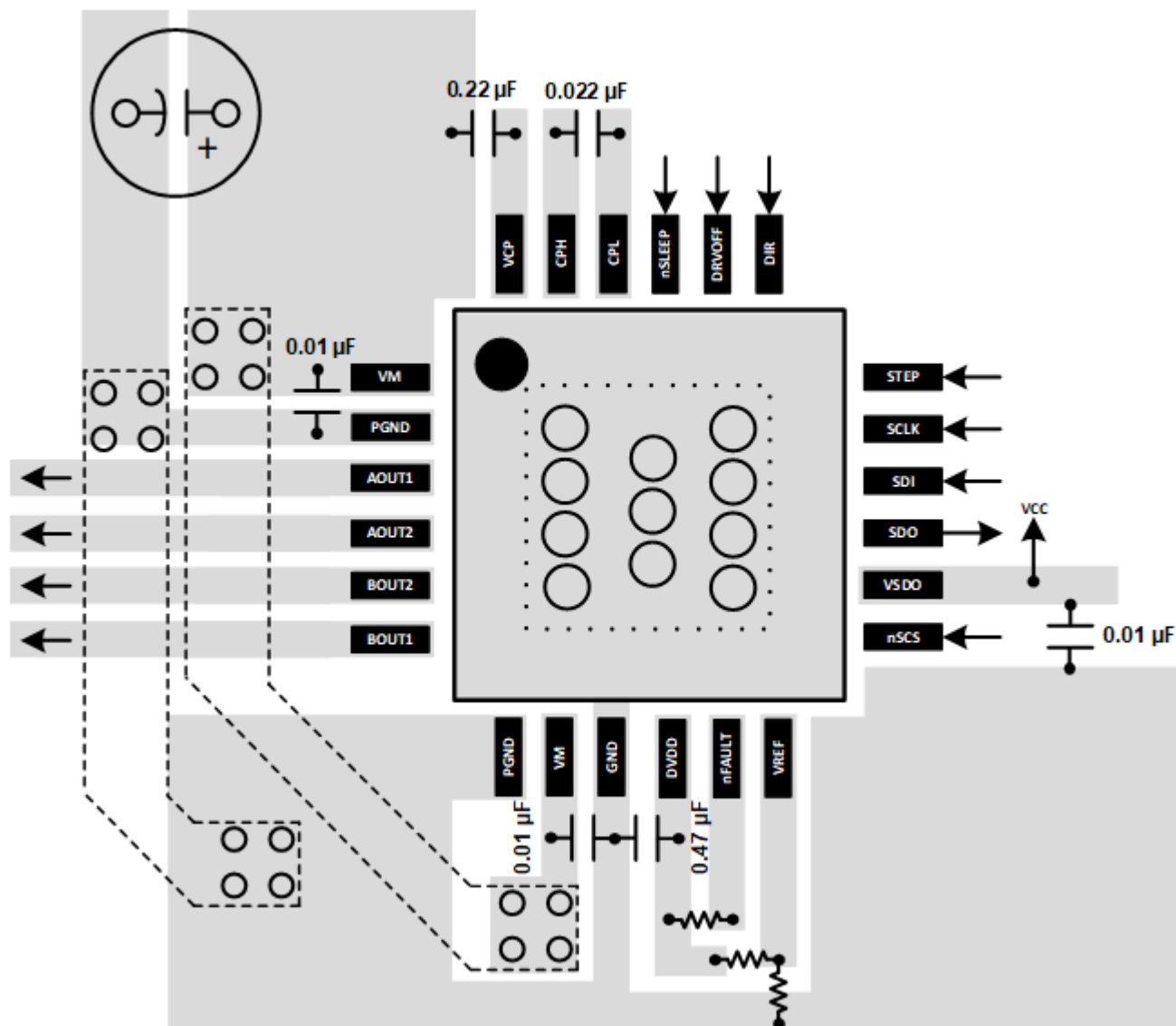
図 10-1. QFN の推奨レイアウト
