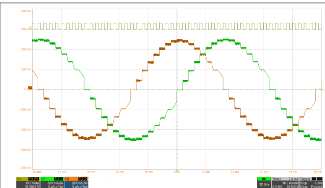
図 8-3. 低速 - 低速減衰による 1/8 マイクロステッピング
