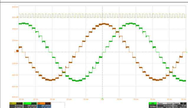
図 8-5. スマート・チューン・ダイナミック減衰による 1/8 マイクロステッピング
