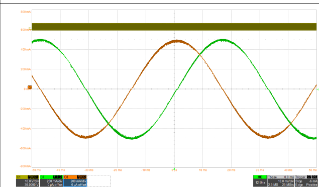
図 8-9. スマート・チューン・ダイナミック減衰による 1/256 マイクロステッピング
