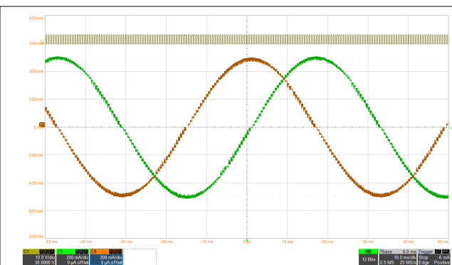
図 8-7. スマート・チューン・ダイナミック減衰による 1/32 マイクロステッピング
