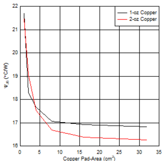
図 8-19. 4 層 PCB の接合部から基板への熱特性パラメータ ( \Psi_{JB} ) と銅面積との関係
