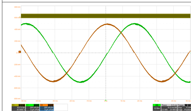
図 8-8. スマート・チューン・リップル制御減衰による 1/256 マイクロステッピング
